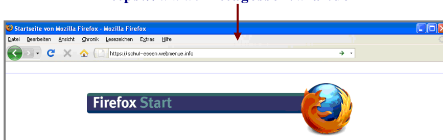
Abb. 2 Internetbestellsystem laden
