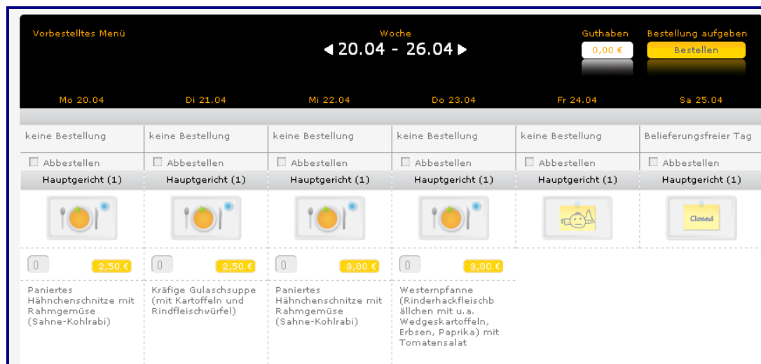
Abb. 1 Internetbestellsystem WebMenü
